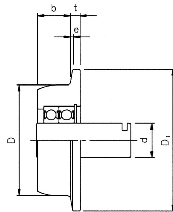
従動輪
