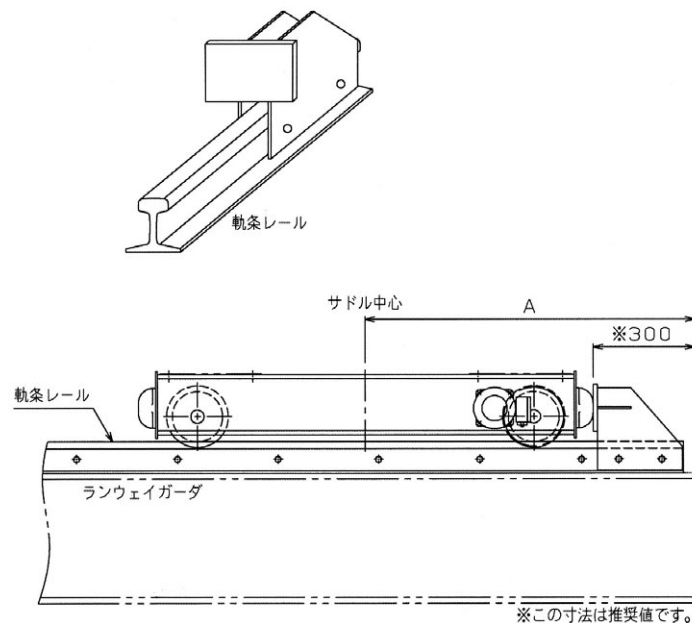
TCS形走行レール用ストップパ
