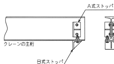
図8 クレーンの主桁用ストップパ
