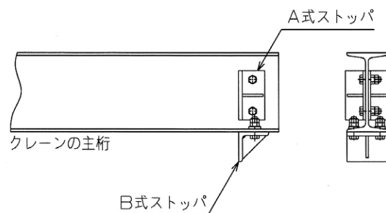
図16 クレーンの主桁用ストップ
