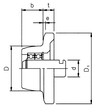
従動輪
