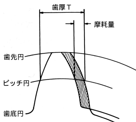
歯車の摩耗説明図
