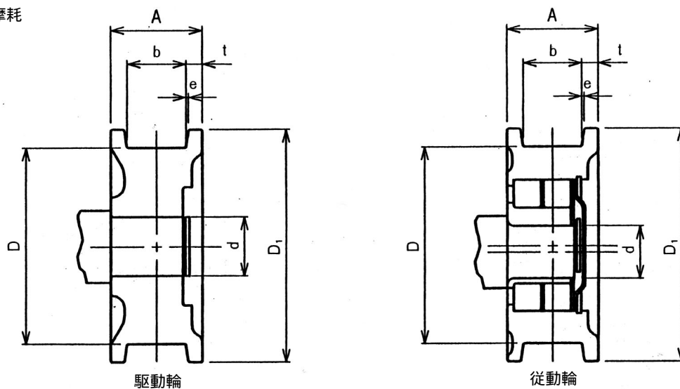
附図2 (2.8、3tダブルレール形横行車輪)
