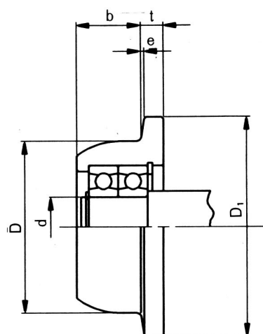
従動輪
