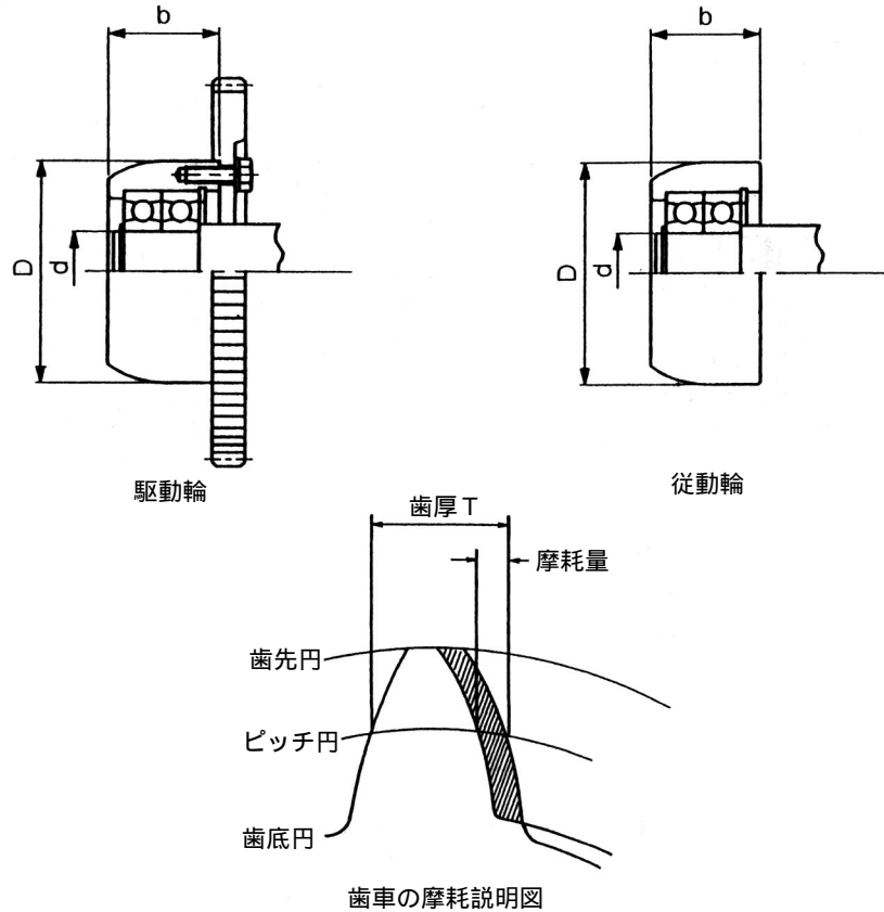
附図1 (Cタイプ)(1、2、2.8、3t用普通形、ローヘッド形横行車輪)
